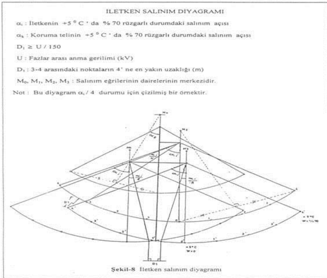
Şekil-8 İletken salınım diyagramı
